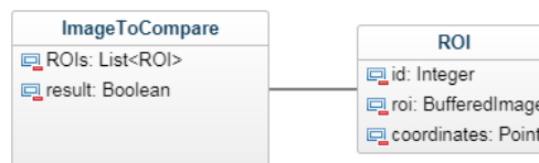
Fig. 12. Objetos ImageToCompare y ROI
